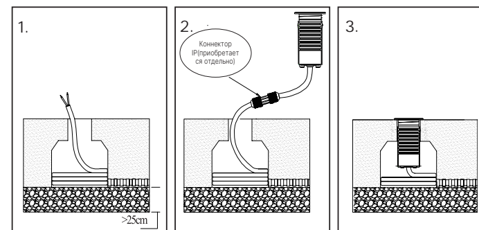
Монтажный стакан MS1
